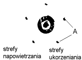
Rys. 6. Przykład ekologicznego zabezpieczenia drzewa z bryłą korzeniową na placu składowym (wg [10])
